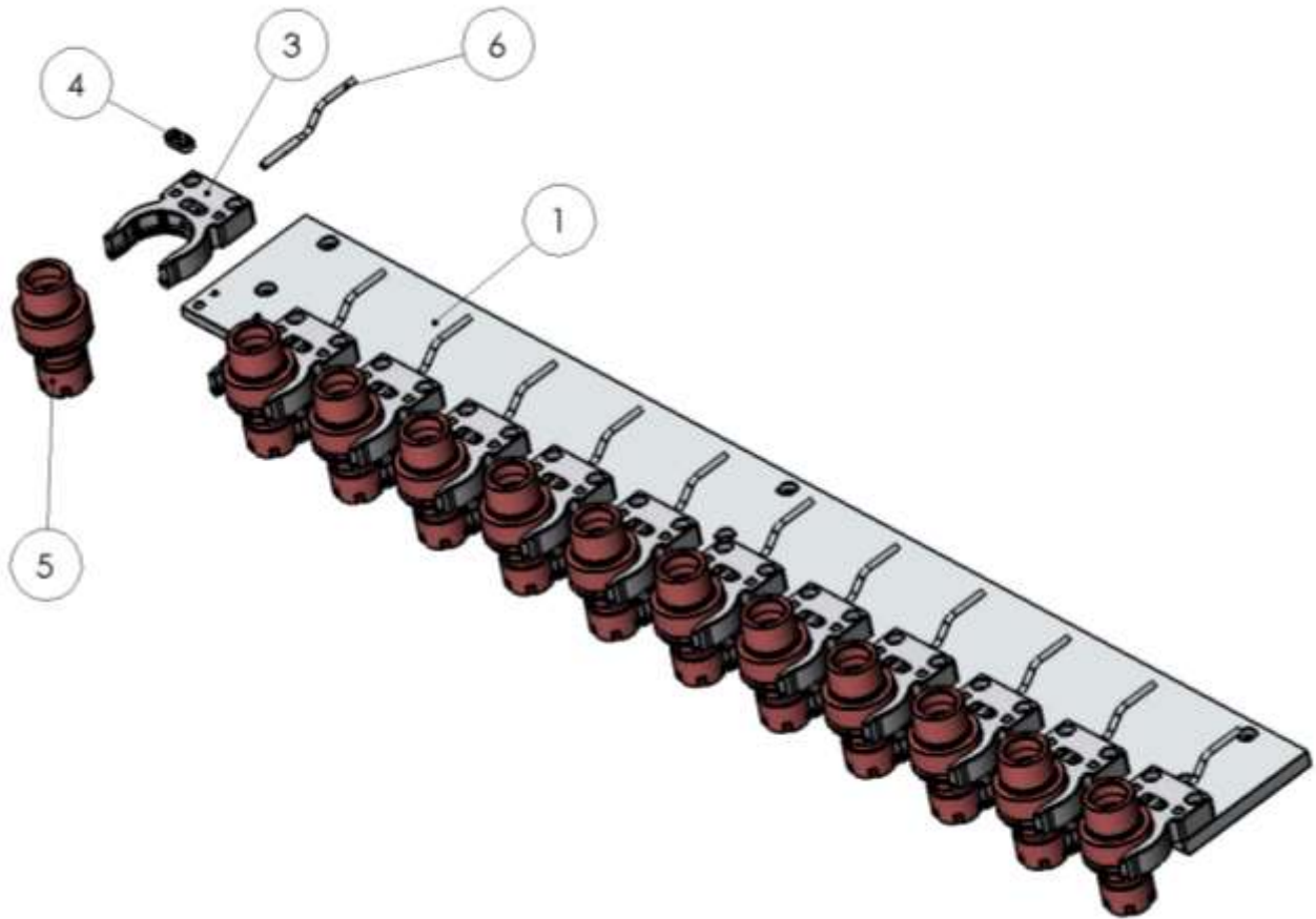
Abbildung 2: Dreheinheitbox (510-1109-0011)
